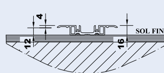
Posé sur sol fini
