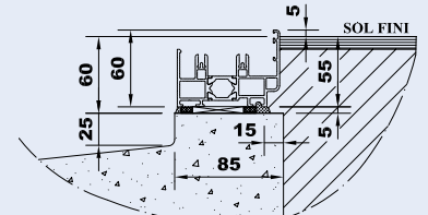
Encastré ouverture extérieure
