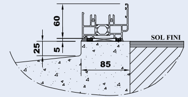
Encastré ouverture extérieure
