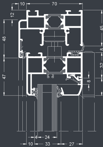
COUPE VERTICALE HAUTE
