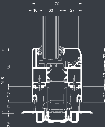
COUPE VERTICALE BASSE avec seuil plat
